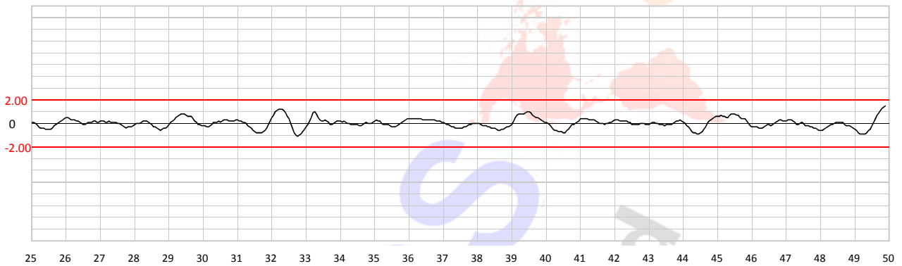
2m Gauge
